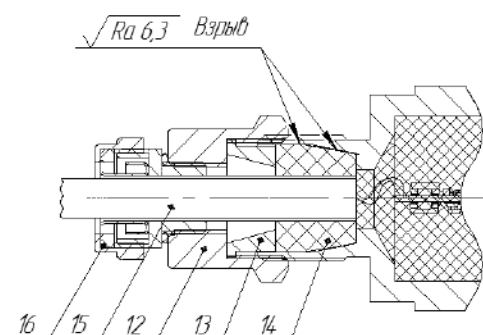
Вариант с устройством крепления металлорукава
