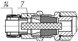
д) кабельный ввод с устройством крепления металлорукава. Остальное – см. а) кабельный ввод по умолчанию
