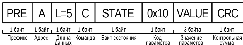
Рисунок 2.5 - Пример пакета байта состояния при включенном режиме ускоренного обмена
