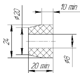
Кольцо уплотнительное поз.14 в свободном состоянии
