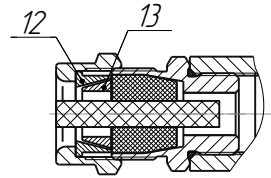
в) кабельный ввод с устройством крепления бронированного кабеля. Остальное – см. а) кабельный ввод по умолчанию.
