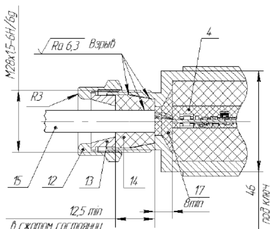
Вариант с устройством крепления металлорукава
