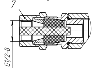
д) кабельный ввод с устройством крепления трубы. Остальное – см. а) кабельный ввод по умолчанию.
