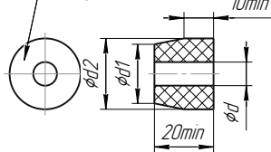
д) кабельный ввод с устройством крепления трубы. Остальное – см. а) кабельный ввод по умолчанию.
