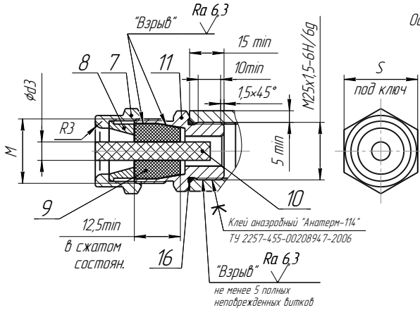
д) кабельный ввод с устройством крепления металлорукава. Остальное – см. а) кабельный ввод по умолчанию
