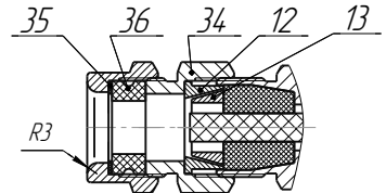
д) кабельный ввод с устройством крепления трубы. Остальное – см. а) кабельный ввод по умолчанию.
