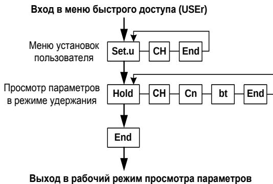
Рисунок 2.2 - Структура меню быстрого доступа
